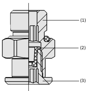
Конструкция системы Ограничители потока SC-SW
